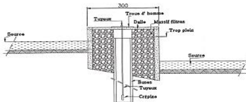
COUPE MUR DE CAPTAGE
